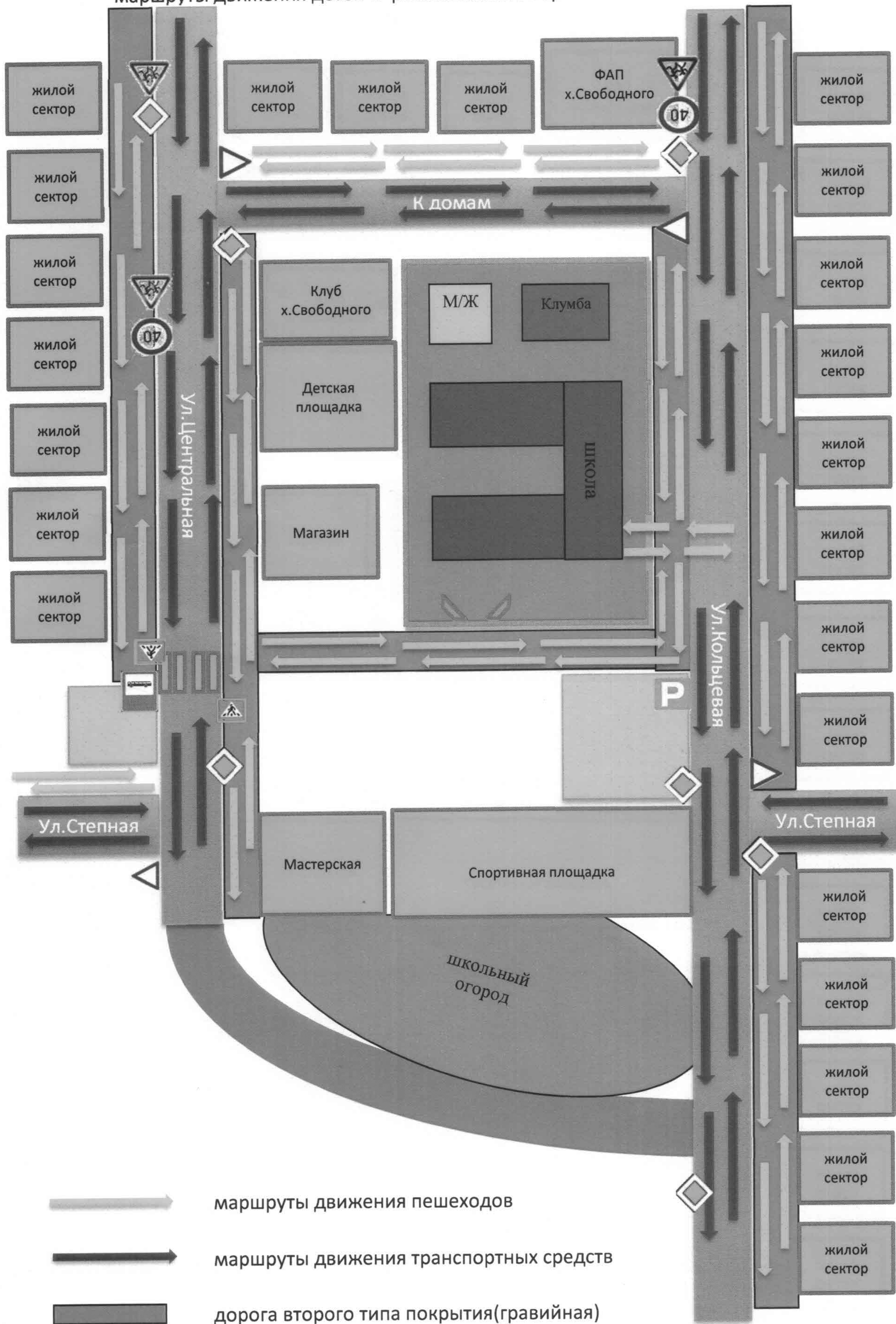
2.Схема организации дорожного движения в непосредственной близости от образовательного учреждения с размещением соответствующих технических средств, маршруты движения детей и расположение парковочных мест
